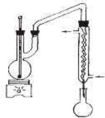
图 3 氟化物蒸馏装置
